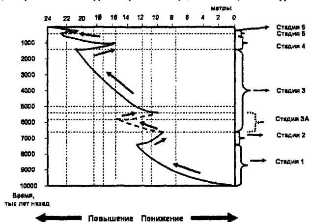
Рис.8 Циклограмма изменений относительного уровня озера Кандрыкул
