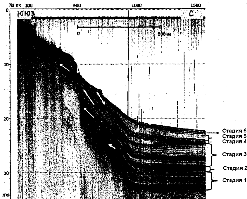
Рис.6 Сейсмоакустический разрез о.Кандрыкуль (профиль 2) с выделенными стадиями развития водоема, стрелки указывают зоны прекращения прослеживания отражений.
