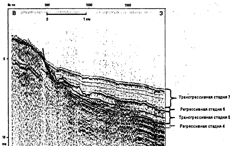
Рис.3 Сейсмоакустический разрез залива Тостубек (профиль 1) с выделенными стадиями развития моря, стрелки-схемы прекращения прослеживания отражений.
