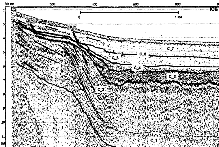
Рис.2 Сейсмоакустический разрез залива Тше-Бас (профиль 2) с выделенными стадиями развития моря, стрелками указано направление трансгрессий и регрессий моря
