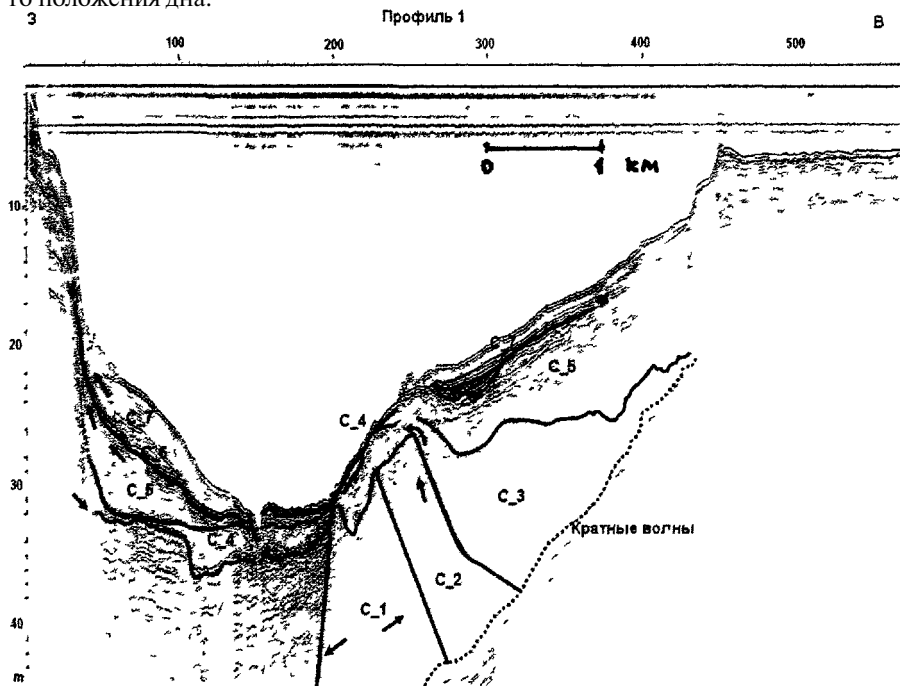
Рис 5 Сейсмоакустический разрез Западно-Аральской котловины с выделенными стадиями (C_1-C_7) развития моря, стрелки указывают зоны прекращения прослеживания отражений
