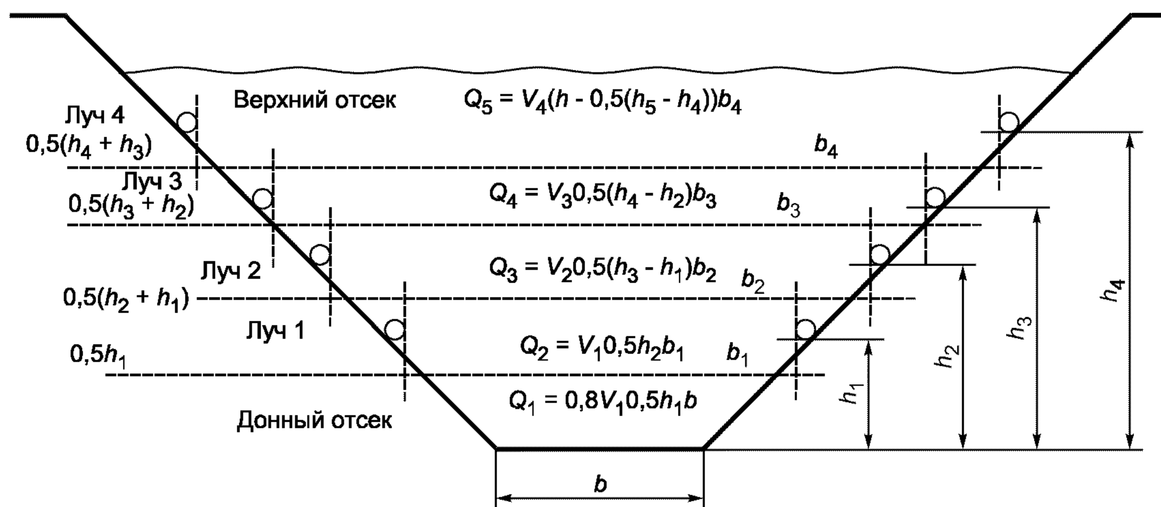
Рисунок 3 — Пример расчета расхода методом послойных сечений
