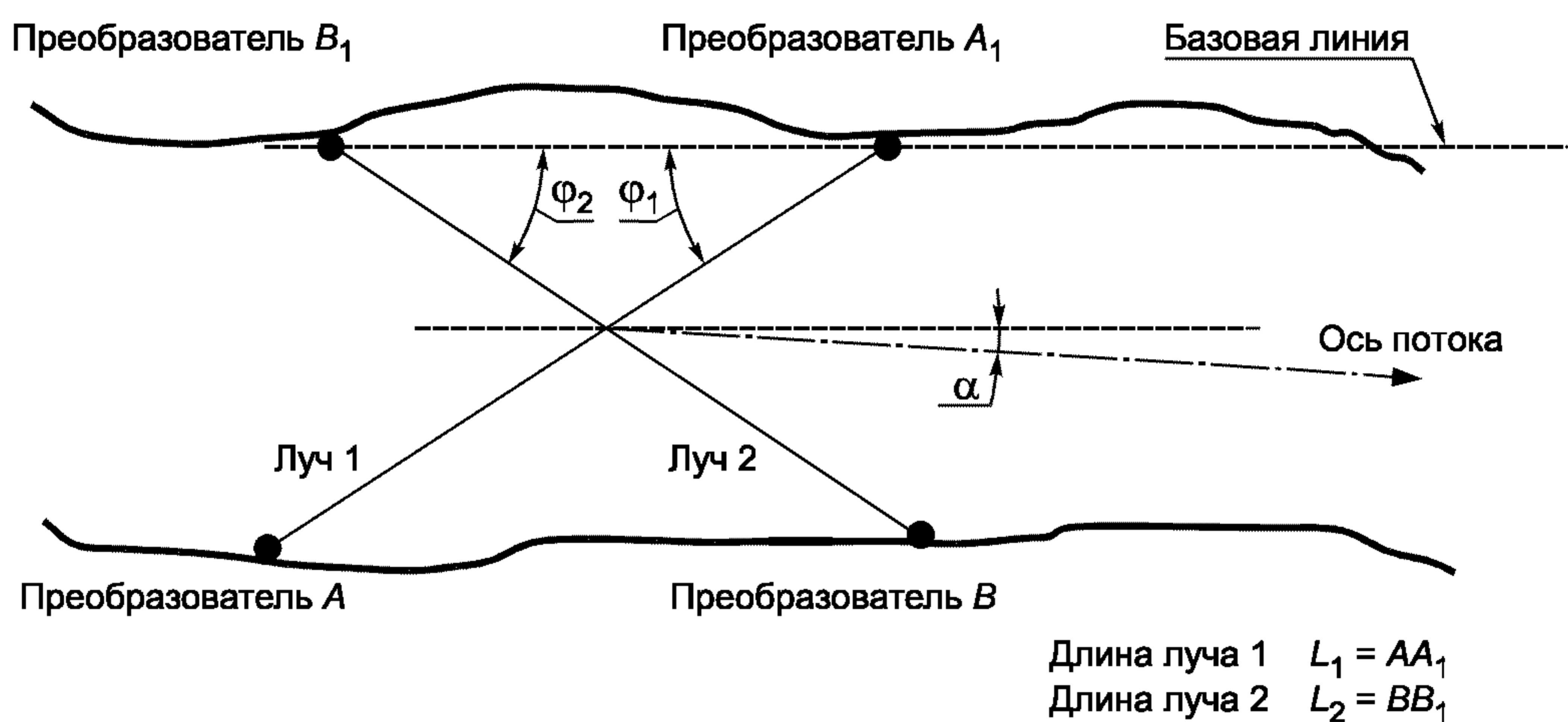
Рисунок 1 — Схема расположения преобразователей с пересекающимися лучами
