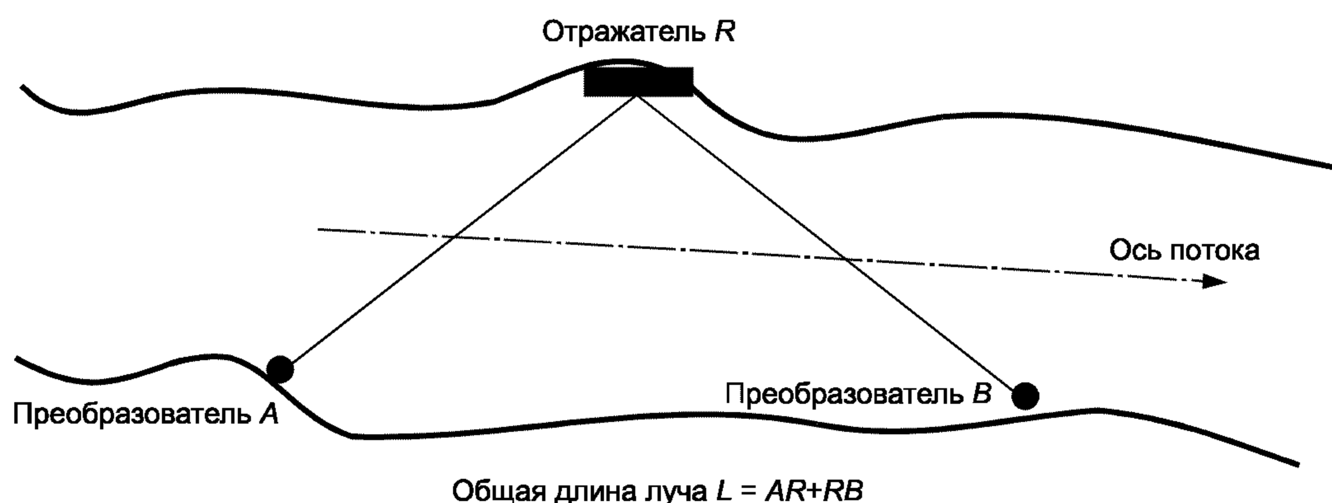
Рисунок 2 — Схема расположения преобразователей с отражением лучей
