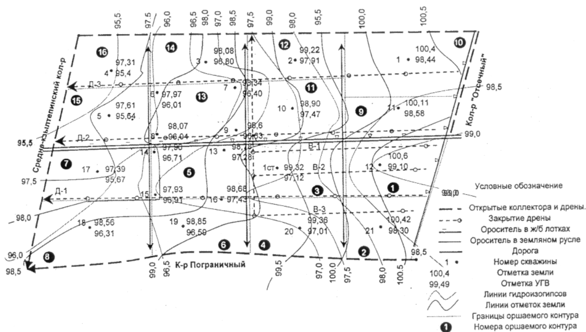
Рис. 4. План-схема и карта гидроизогипс фермерского хозяйства «Азизбек-1» Ахунбабаевского района по состоянию на 07.08.04.
