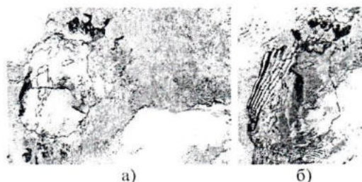
Р и с. 5. а) Снимок за 19.11.12, terra.721.1km; б) снимок за 17.11.12, terra.721.1km
