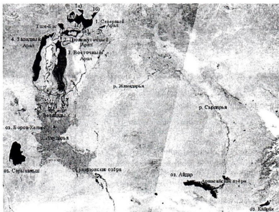
Р и с. 1. Снимок района Приаралья, полученный 09.10.10 со спутника TERRA; 1а) – залив Бутакова, 1б) – залив Сары-Чеганак, 1в) – пролив Берга, 1г) – залив Нессельроде, 1д) – залив Шевченко. Цифрами 5 обозначены ветланды; 5а) – Муйнак-Рыбачье, 5б) – Джилтыр-Бас-2, 5в) – Судочье, 5г) – Междуречье, 5д) – Джилтыр-Бас
