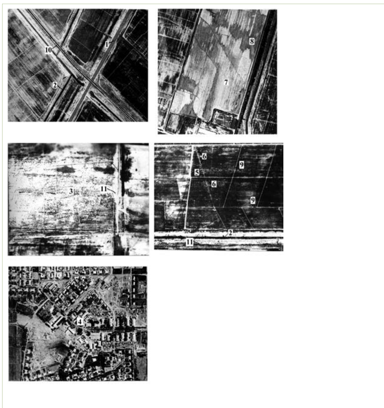
Рис. 12.8. Выделение на аэрофотоснимках некоторых объектов: 1- каналы, 2 – коллекторы, 3 – неудобья, 4 – населенные пункты, 5 –расположение закрытого дренажа (видны смотровые колодцы (6)); 7 – свежевспаханное поле и поливы на нем (8); 9 – ок-арыки; 10 – дороги шоссейные; 11 – дороги грунтовые
