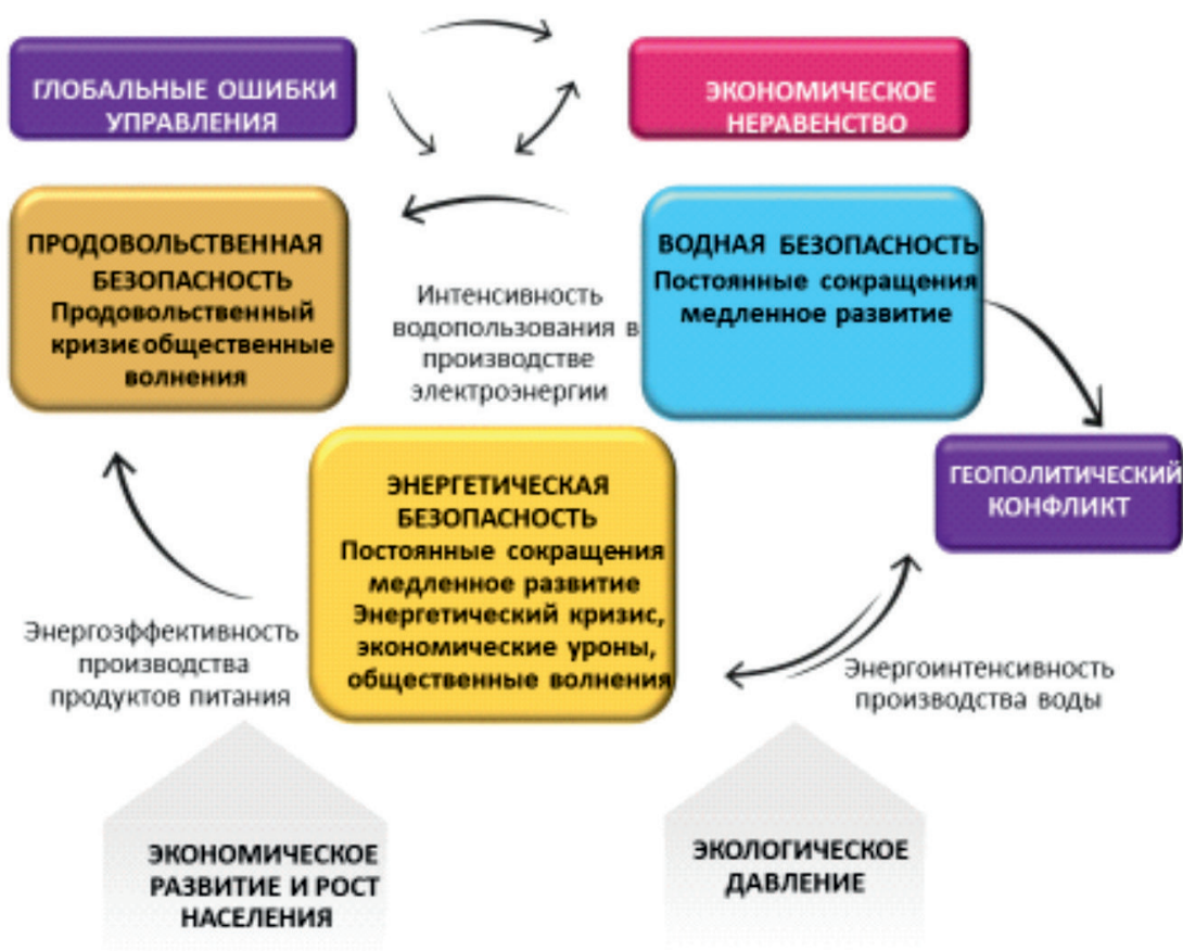
Рисунок 3. Взаимосвязь водной, энергетической, продовольственной безопасности
